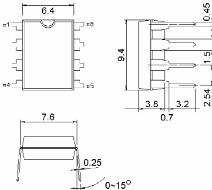
DIP8 封装尺寸
